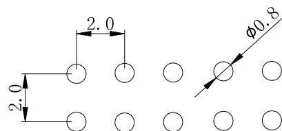
P.C.B Hole Layout
