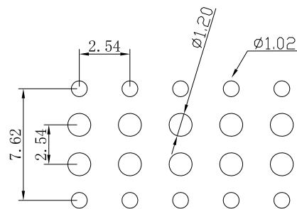
P.C.B Hold Layout
